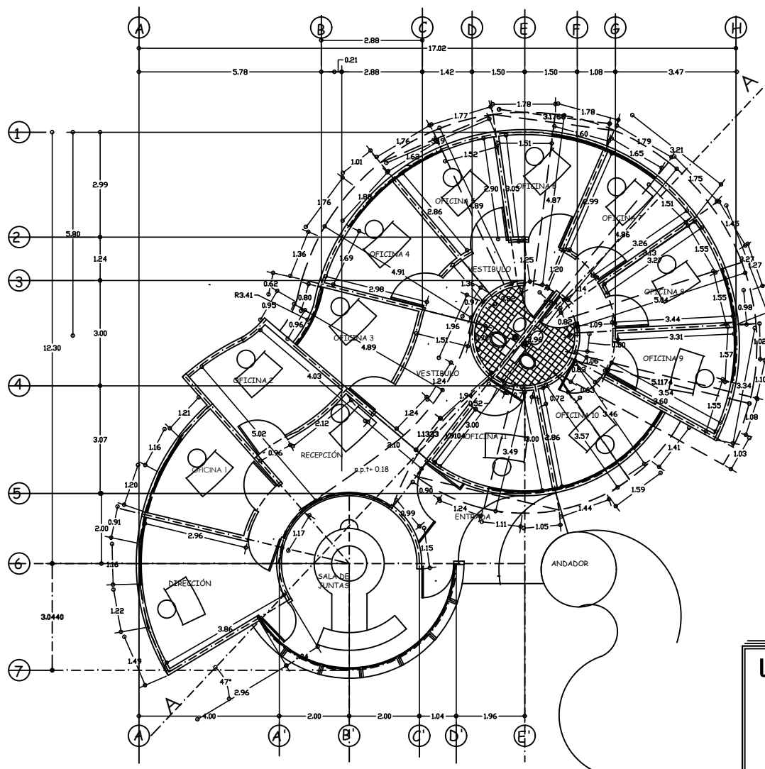
PLANTA ARQUITECTONICA
