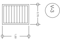
V-3 aluminio anodizado color negro 2° cristal flocado 4mm labada en perlas
